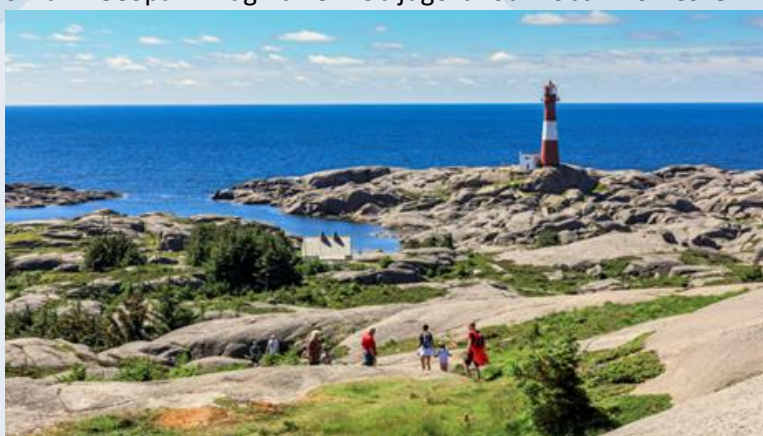
Slike 8: Svetilnik Eigerøy s Severnim morjem v ozadju je v značilnem anortozitnem okolju. (foto: arhiv Geopark Magma)
